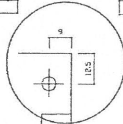
B部 拡大図 S=1/1
