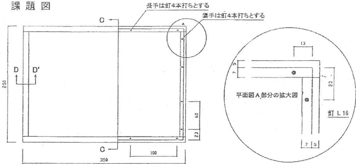
平面図 S=1/3
