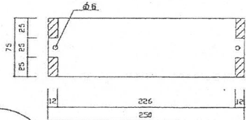
妻手側面図 S=1/3
