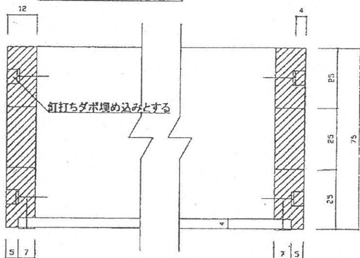
B部 拡大図 S=1/1
